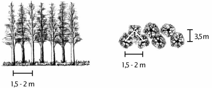
Figura 8: Cortina doble de álamo criollo. Vista de frente(izq), vista en planta (der)
