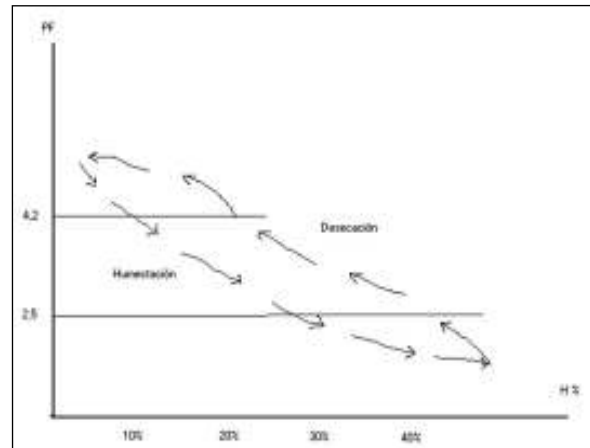
Figura 4. Curva de histéresis que muestra la relación tensión humedad de un suelo por la vía de la humectación o desecamiento.
