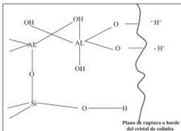
Figura 7. Carga negativa en el borde de las arcillas. En este caso los oxígenos serían las cargas negativas (insatisfechas). A pH superiores a 7 los hidrógenos están débilmente retenidos y pueden ser fácilmente intercambiados por otros cationes. Adaptado de Darwich, 1998.
