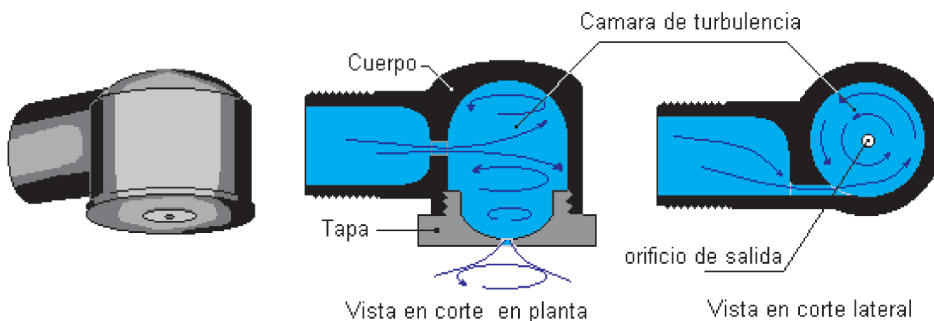
FIGURA III 28: Vista y corte de una pastilla gran angular
