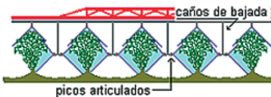
FIGURA IV.39: Esquema de una aplicación con tubos de bajada y vista de un pico múltiple articulado orientable (derecha)
