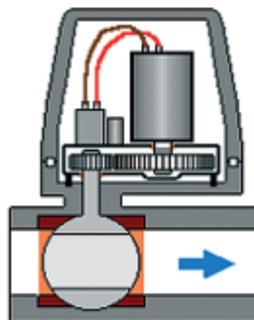
FIGURA IV. 56: Esquema del regulador de presión caudal.
