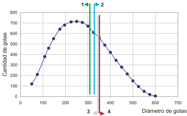
Figura II.8: Espectro de pulverización. Referencias: 1) ( D_{\bar{x}} ); 2) ( DV_{\bar{x}} ); 3) ( DV_{0,5} ); 4) ( DM_s )
