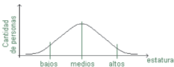
Figura II.4: Distribución Normal
