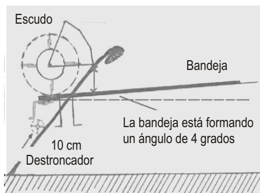
Figura 7: Regulación de la posición del escudo del destroncador.
