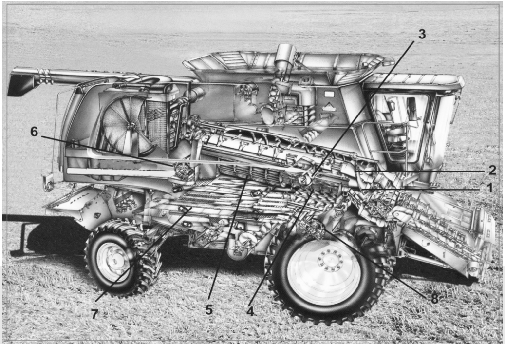
Figura 24: Cosechadora de flujo axial: 1) Cono de entrada; 2) Rotor; 3) Barras batidoras; 4) Cóncavos de trilla; 5) Cóncavos de separación; 6) Despajador de descarga; 7) Zarandas de limpieza; 8) Turbina de aire.
