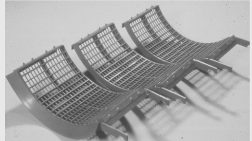
Figura 26: Cóncavos de trilla de la cosechadora axial (generalmente dispuestos en tres tramos)
