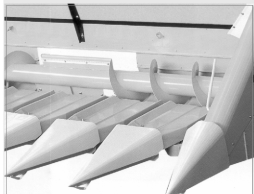
Figura 21: Detalle de los puntones de recolección agudos
