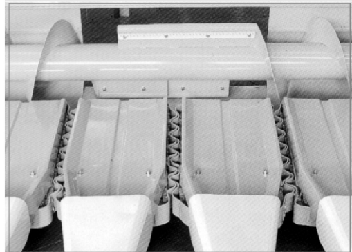
Figura 20: Detalle de los puntones de recolección agudos, batea de captación y cadena de guía y transporte.
