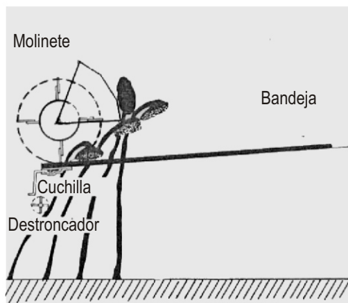
Figura 6: Funcionamiento del cabezal giratorio.
