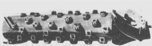
Figura 25: Rotor de la cosechadora axial.
