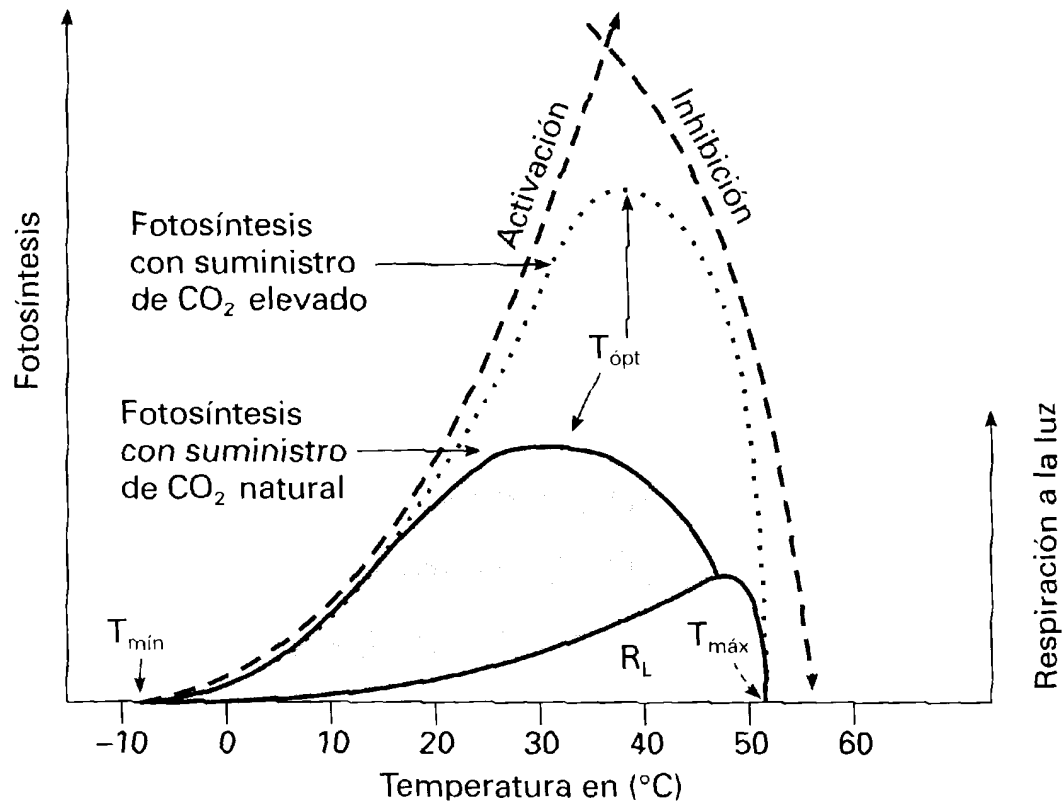
Figura 13-12. Respuestas a la temperatura de la fotosíntesis a niveles de CO_2 ambiental y elevado, en plantas C_3 . T_{opt} : temperatura óptima para la fotosíntesis; T_{min} : límite inferior de temperatura; T_{máx} : límite superior; R_L : estimación de la respiración a la luz (principalmente fotorrespiración). (Adaptado de Larcher, W. Physiological Plant Ecology . Springer-Verlag, 1995.)
