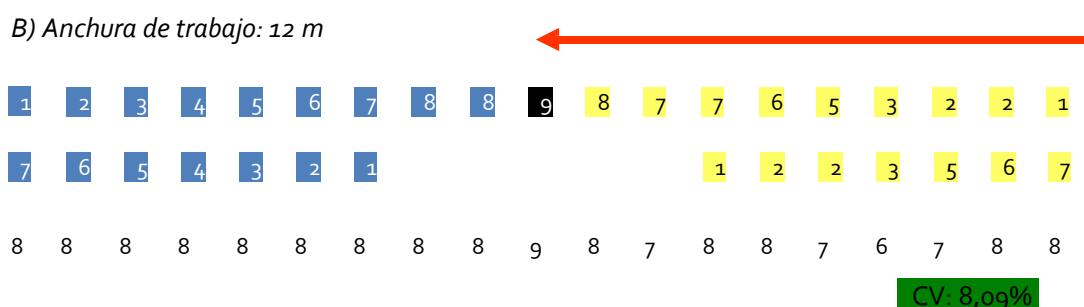
Figura 12: Coeficientes de variación de dos aplicaciones con el mismo perfil de distribución (fila superior) y diferente ancho de trabajo trabajando en forma alternada (ida y vuelta). En la medida que crece el ancho de trabajo también lo hace el coeficiente de variación
