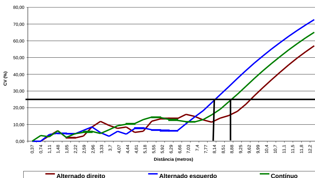
Figura 15: Gráfico de Coeficiente de variación en función de la distancia entre pasadas y de la forma de trabajo. Para no superar el CV de 25% las pasadas se deben distanciar 8,88m en continuo u 8,14m en Alternado
