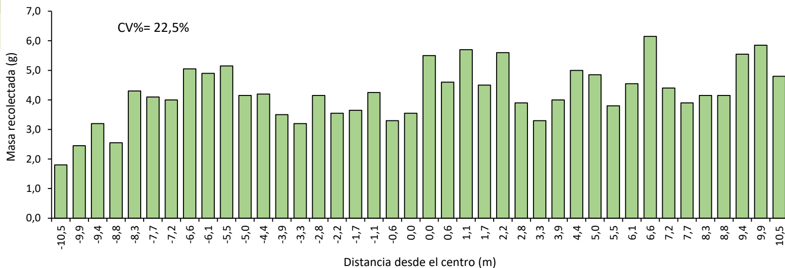
Figura 13. Distribución de urea en el ancho de labor de Fertilizadora RoGator AirMax 1300 R1.
